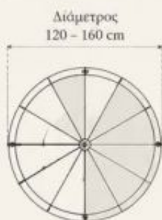
Ελικοειδής σκάλα με κεντρικό άξονα
